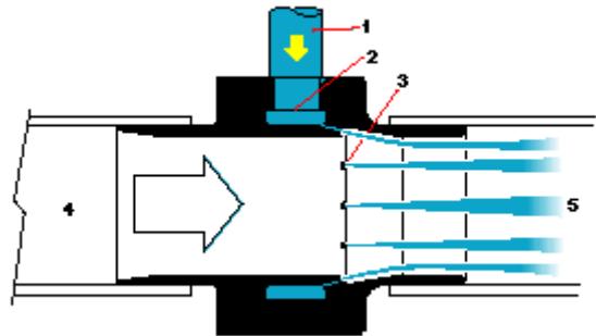
Werkingsprincipe
